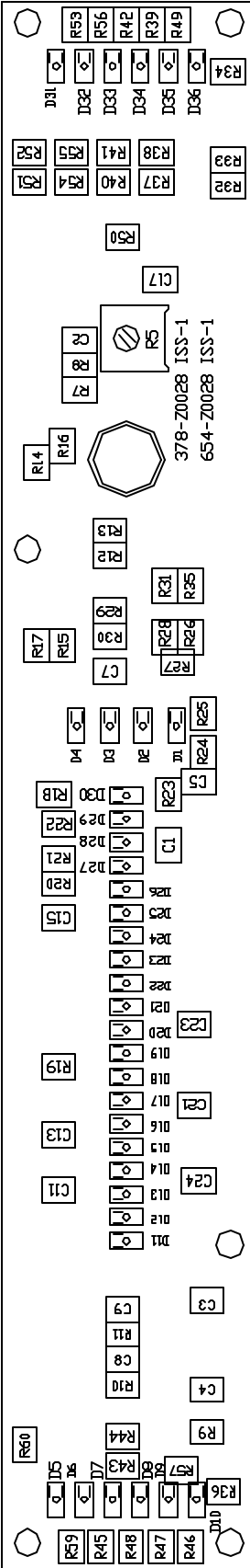
654Z0028.DWG
