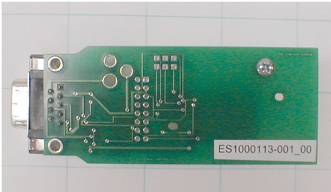
PCB Bottom
