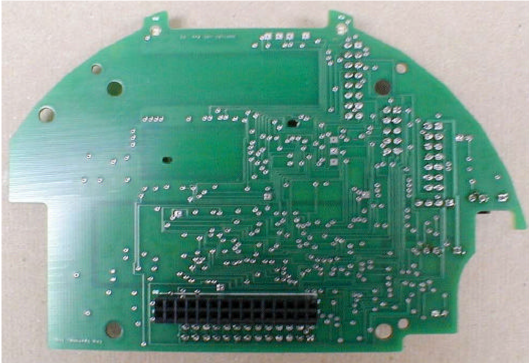
Module Bottom
