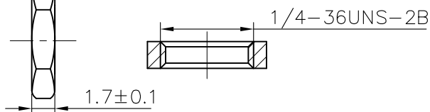
Nut
