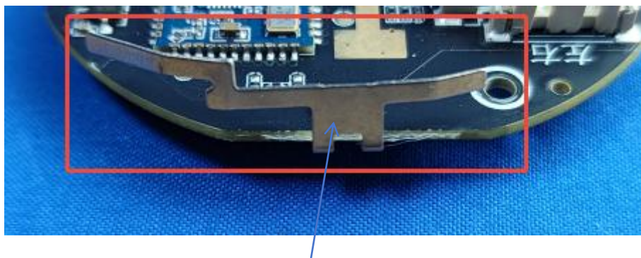
PIFA antenna
