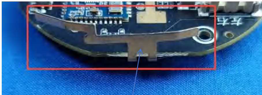
PIFA ANT
