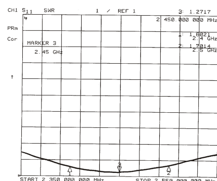
VSWR
