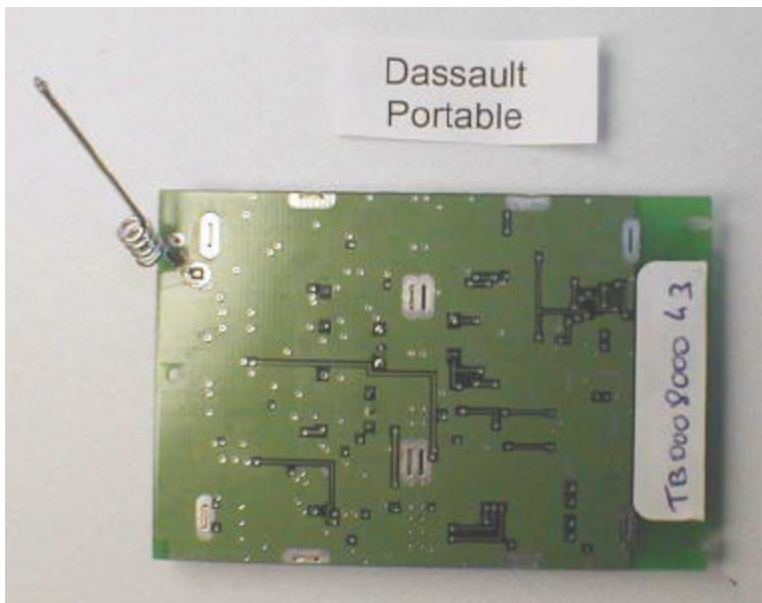
RF Module PCB Bottom
