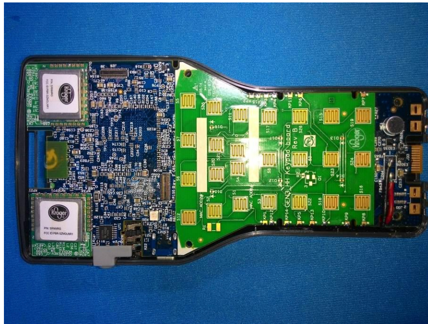
EUT without Keypad
