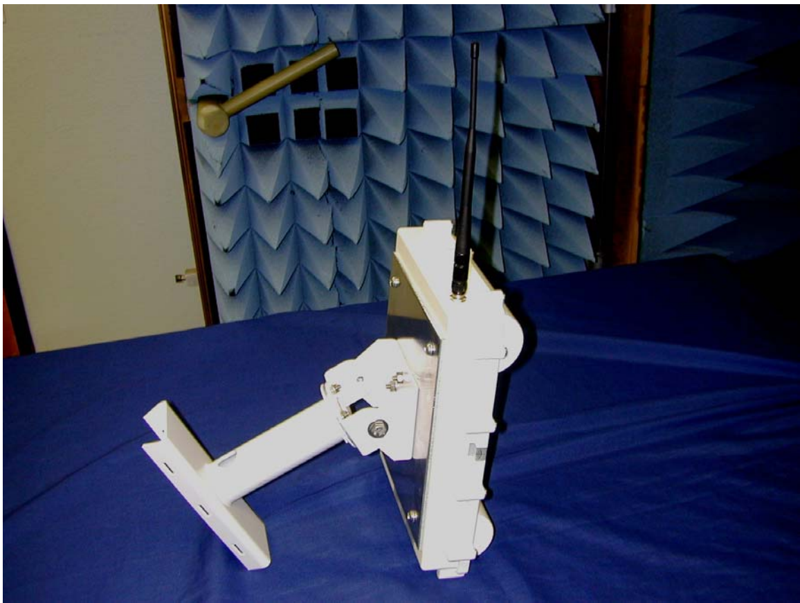
Left EUT
