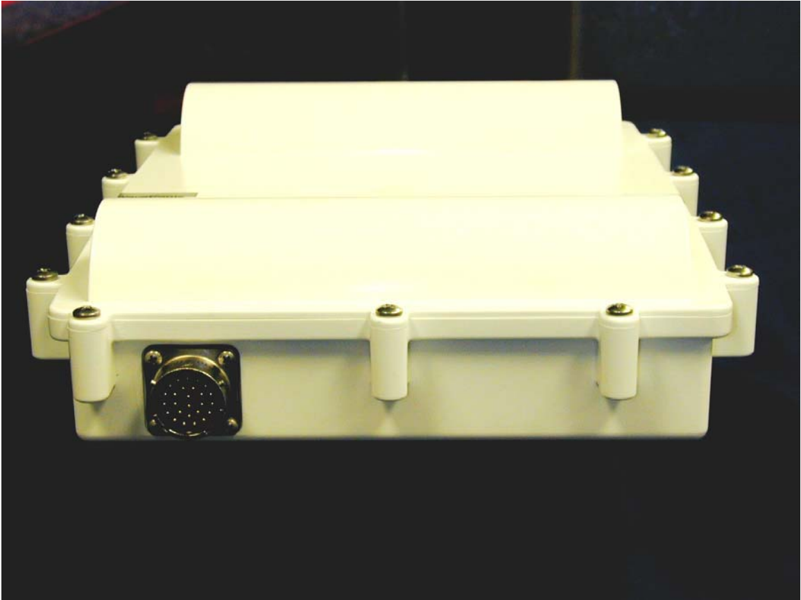
Bottom EUT
