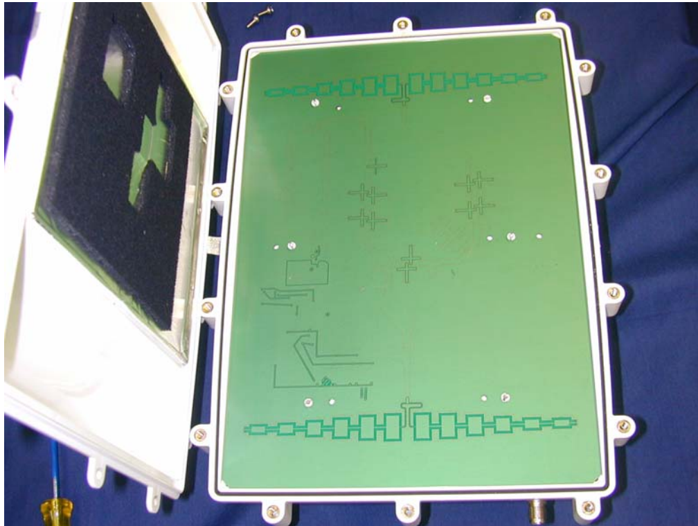
Int. Antenna
