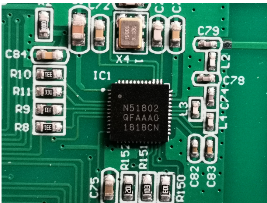
EUT –PCB-1 Bottom Chip View-2
