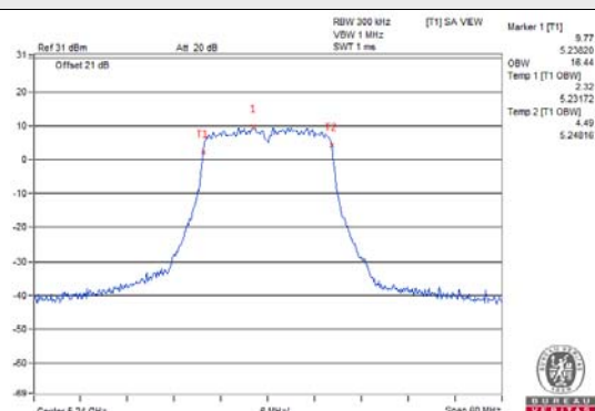
802.11a / Chain 3 / CH 48
