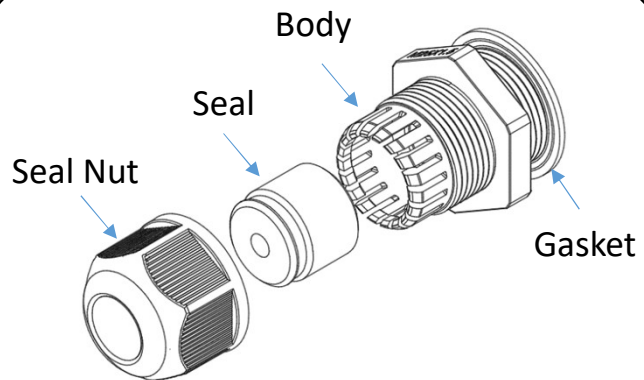
Cable Gland
