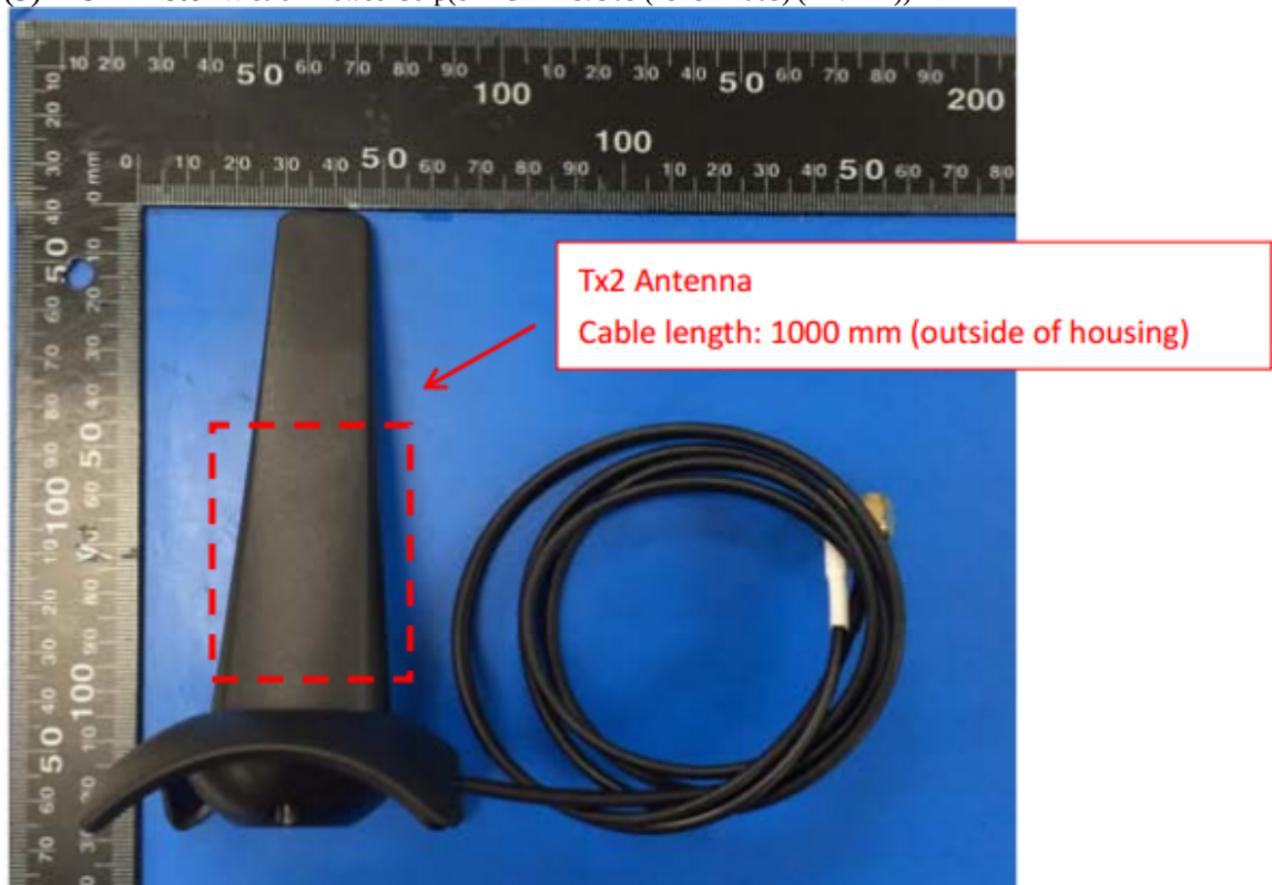
(9) EUT Photo- Wistron Neweb Corp(81XCAA15.G03 (497317-003) ( Tx/Rx2))
