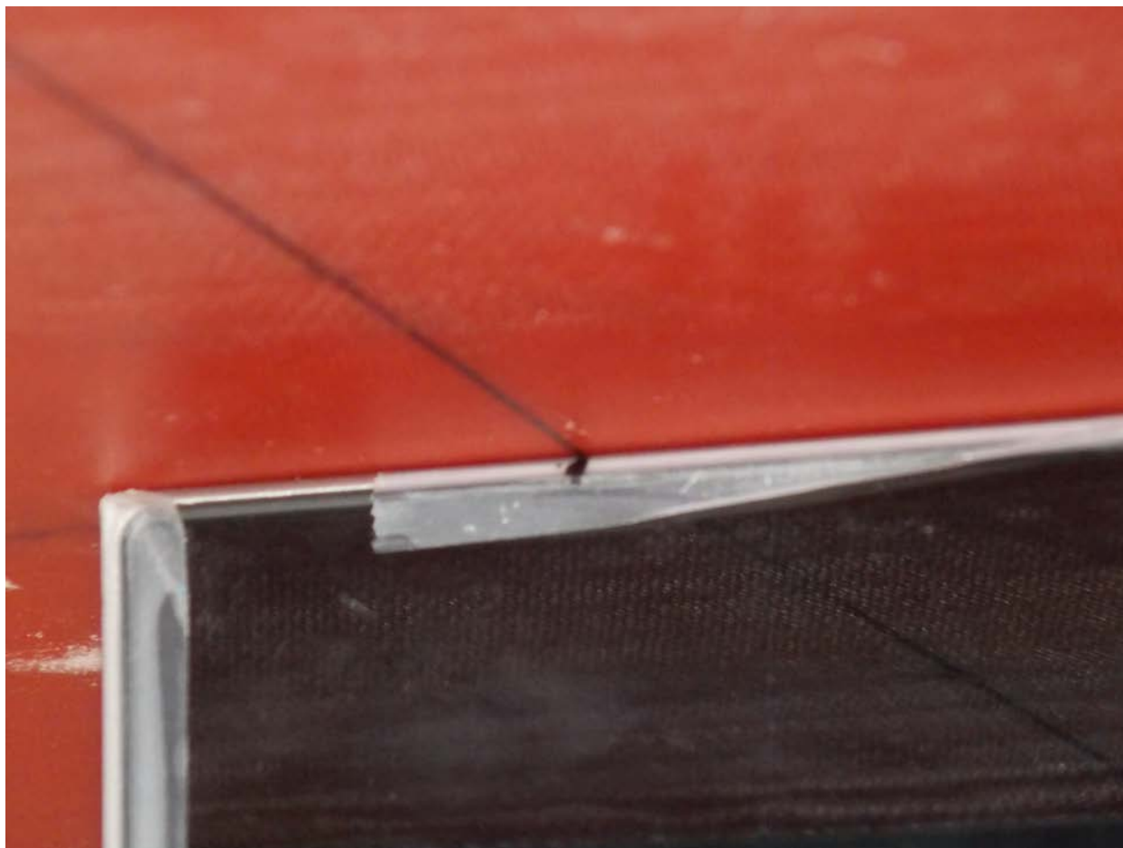
Test Position Tablet Mode Top Edge 0 mm Gap
