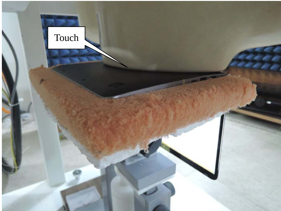
EUT Bottom
