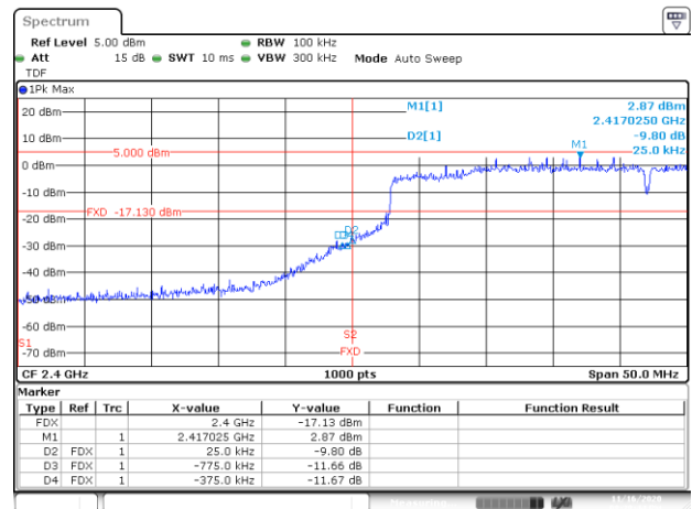
BE-NR, DIV-1, 802.11ax40-HE0, Ch3
