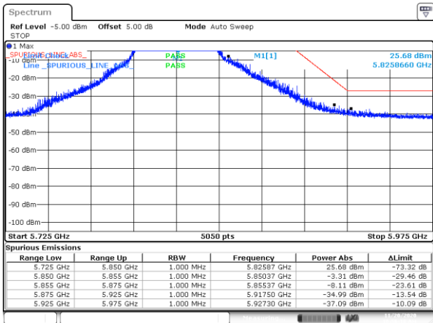
BE-NR-HIGH, DIV 2, 802.11ax20-HE0, Ch165
