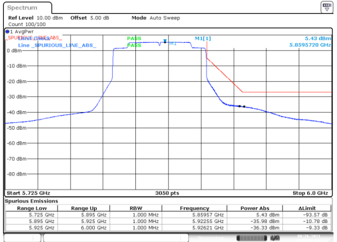
BE-NR-HIGH, MIMO-B, 802.11ax80-HE0, Ch171
