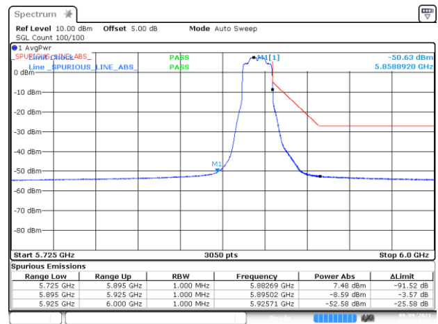
BE-NR-HIGH, MIMO-B, 802.11ax20-HE0, Ch177
