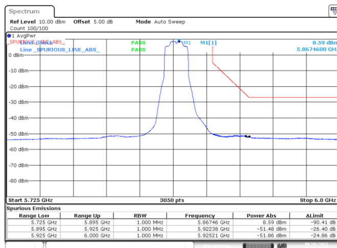
BE-NR-HIGH, MIMO-A, 802.11ax20-HE0, Ch173
