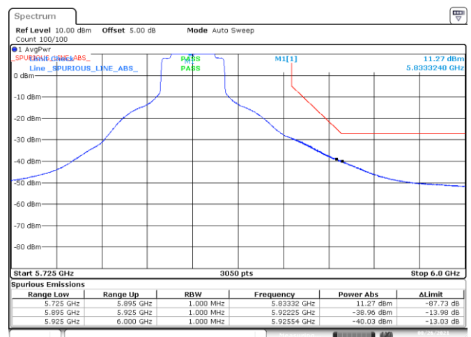
BE-NR-HIGH, MIMO-B, 802.11ax40-HE0, Ch167
