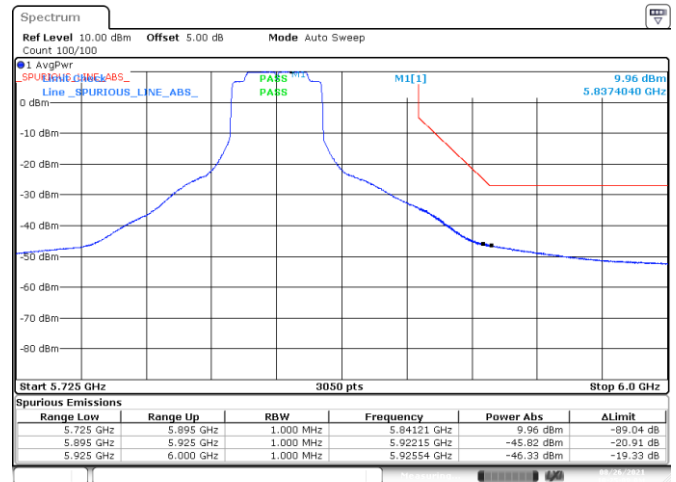
BE-NR-HIGH, MIMO-A, 802.11ax40-HE0, Ch167
