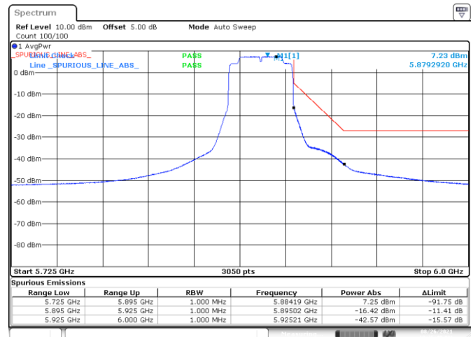
BE-NR-HIGH, MIMO-A, 802.11ax40-HE0, Ch175
