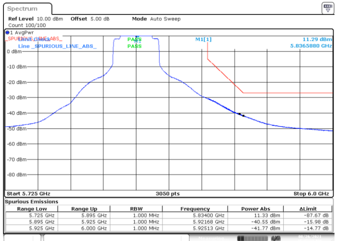
BE-NR-HIGH, SISO-B, 802.11ax40-HE0, Ch167
