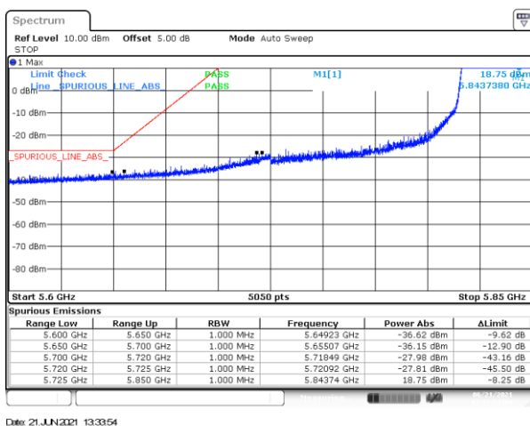
BE-NR-LOW, MIMO-A, 802.11ax80-HE0, Ch171
