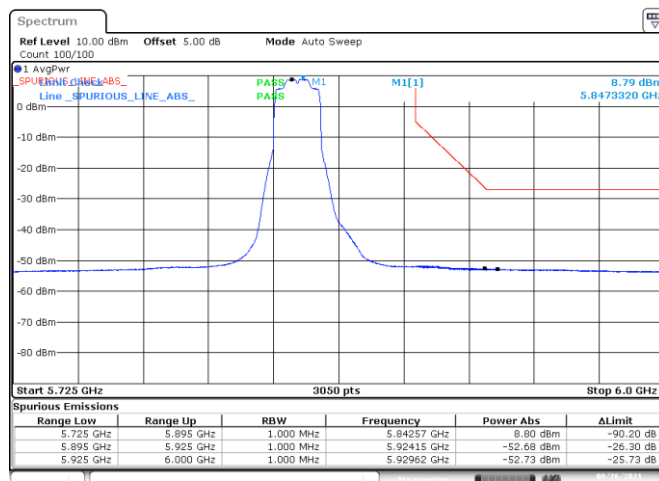
BE-NR-HIGH, MIMO-A, 802.11ax20-HE0, Ch169
