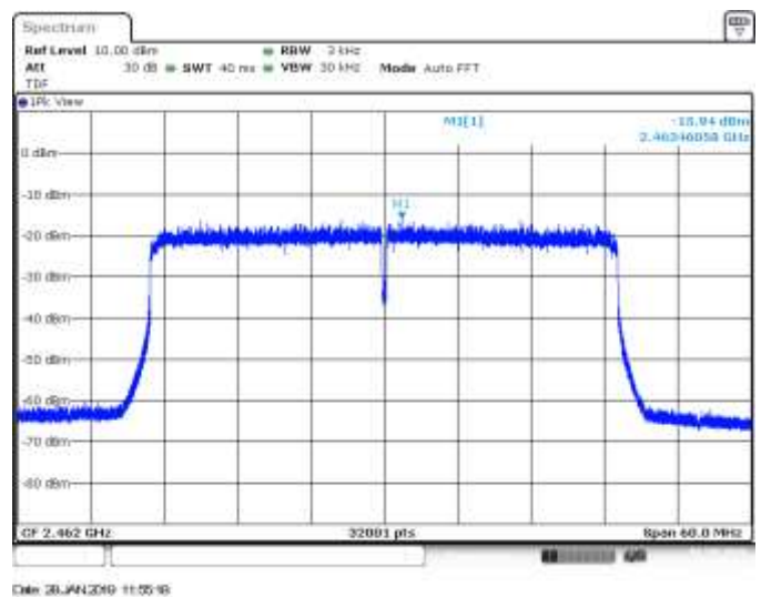
SISO B, CH11, 802.11ax40, HE0, PSD
