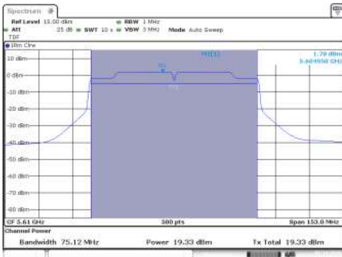
MIMO B, CH122, 802.11ac80, VHT0
