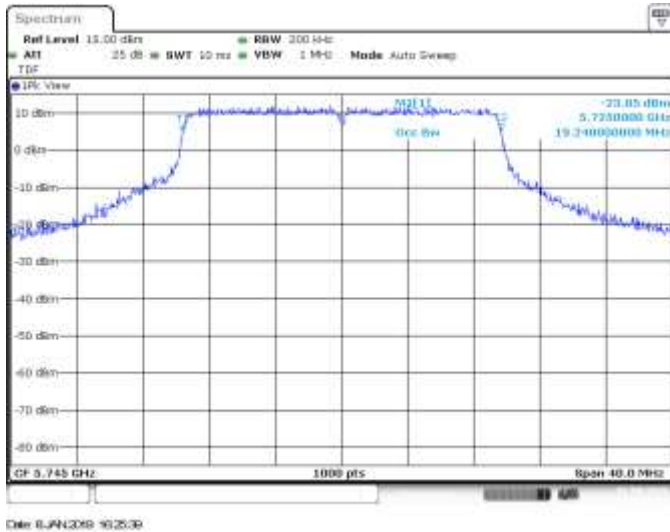
SISO B, CH149, 802.11ax20, HE0, 99% BW
