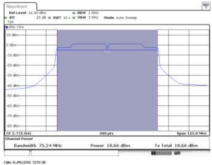
MIMO A, CH155, 802.11ac80, VHT0
