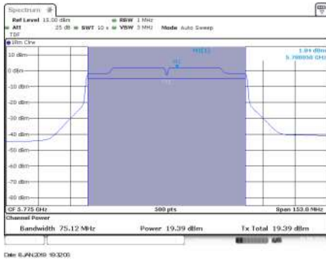
SISO B, CH155, 802.11ac80, VHT0
