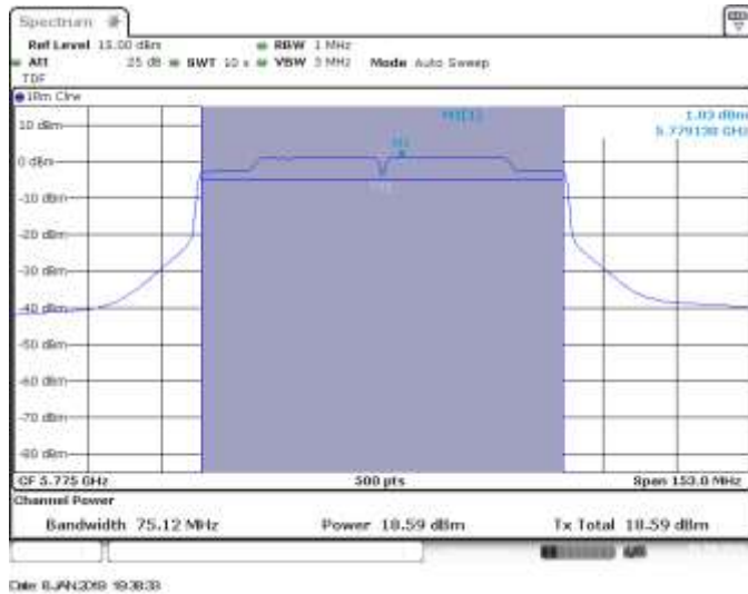
MIMO B, CH155, 802.11ac80, VHT0
