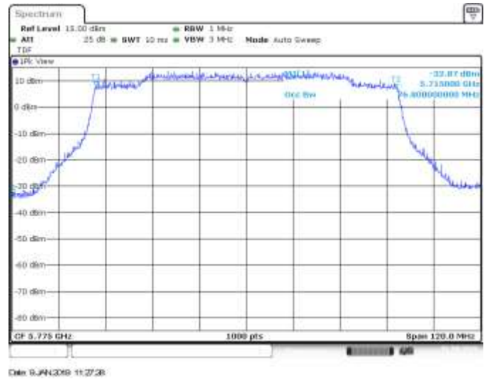
SISO B, CH155, 802.11ax80, HE0, 99% BW
