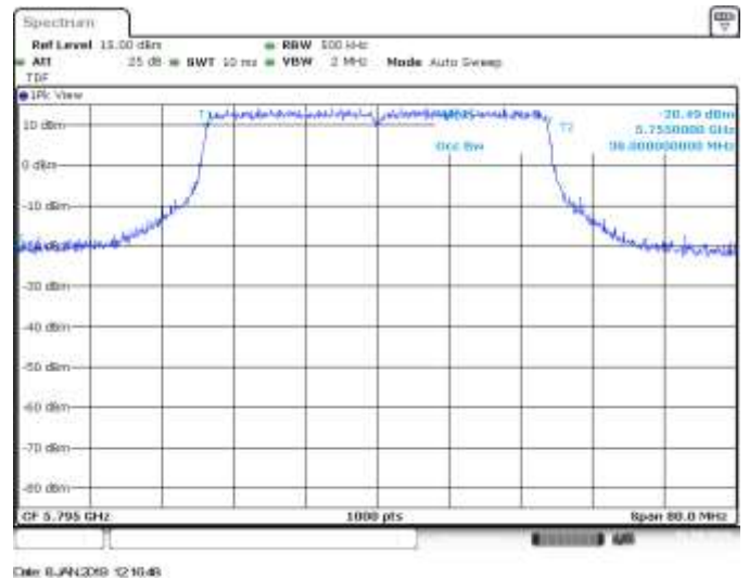
SISO A, CH159, 802.11ax40, HE0, 99% BW
