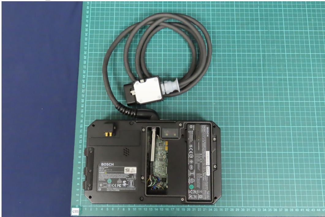
(16) EUT Photo_M/N: 3571-0100-3x (no VCI)
