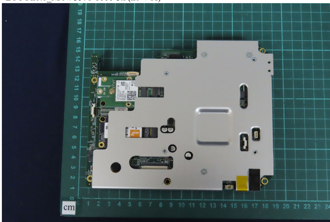
(27) EUT Photo_M/N: 3571-0100-3x (no VCI)
