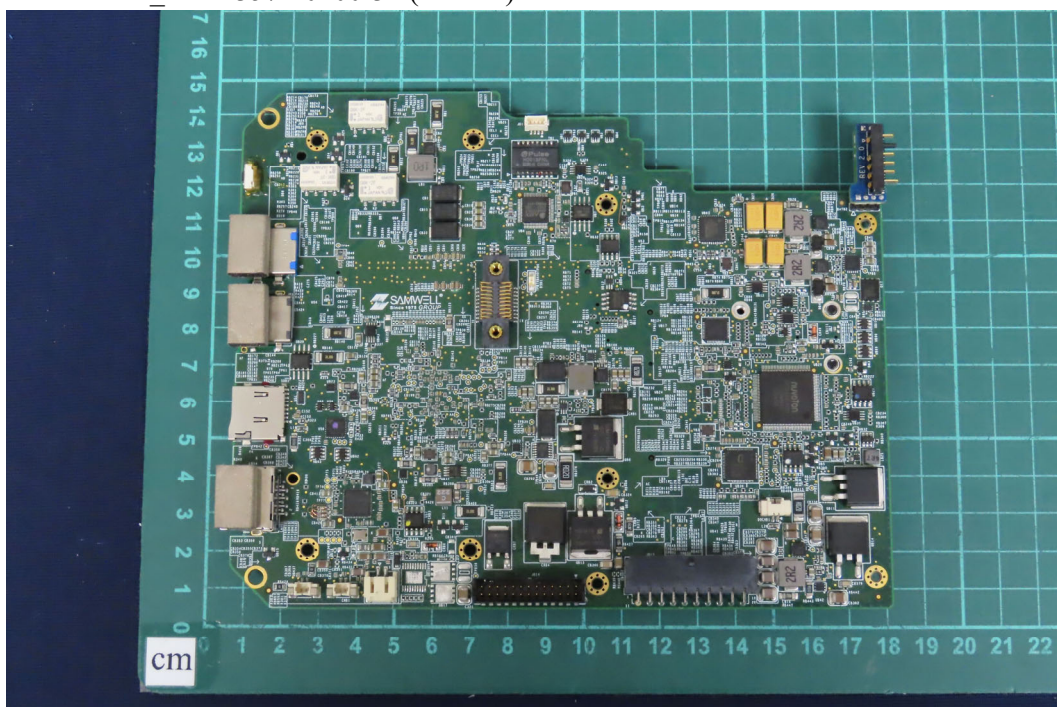
(30) EUT Photo_M/N: 3571-0100-3x (no VCI)
