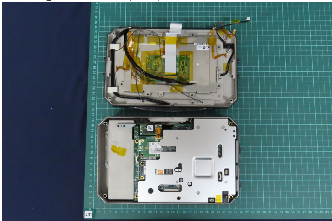
(22) EUT Photo_M/N: 3571-0100-3x (no VCI)
