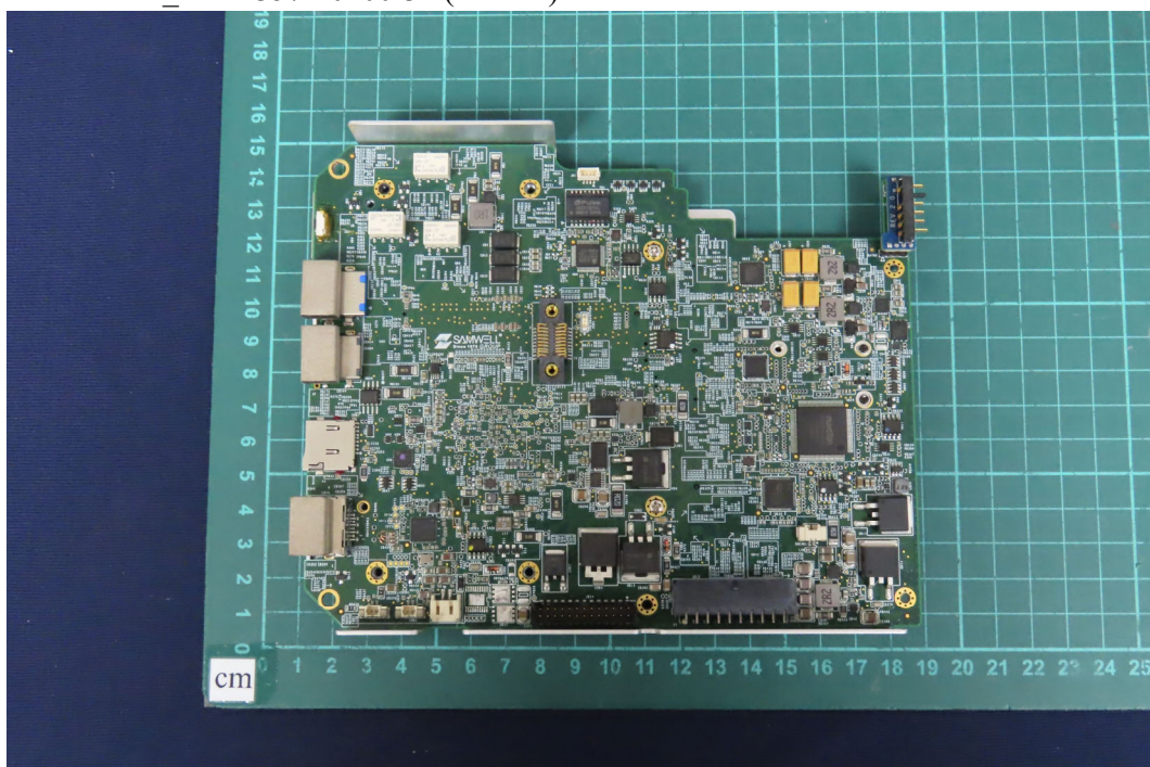
(28) EUT Photo_M/N: 3571-0100-3x (no VCI)
