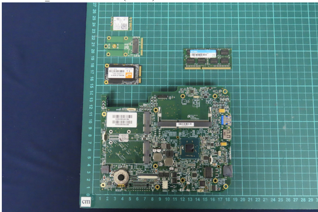
(32) EUT Photo_M/N: 3571-0100-3x (no VCI)
