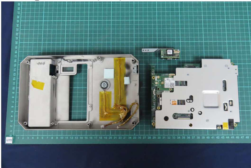
(24) EUT Photo_M/N: 3571-0100-3x (no VCI)
