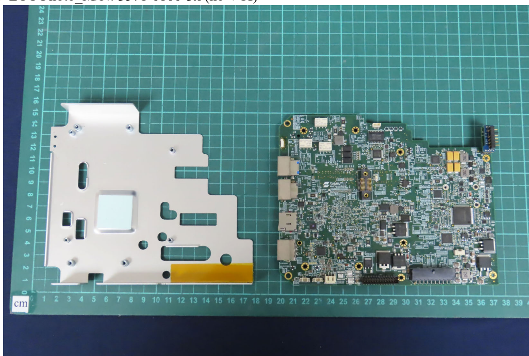
(29) EUT Photo_M/N: 3571-0100-3x (no VCI)
