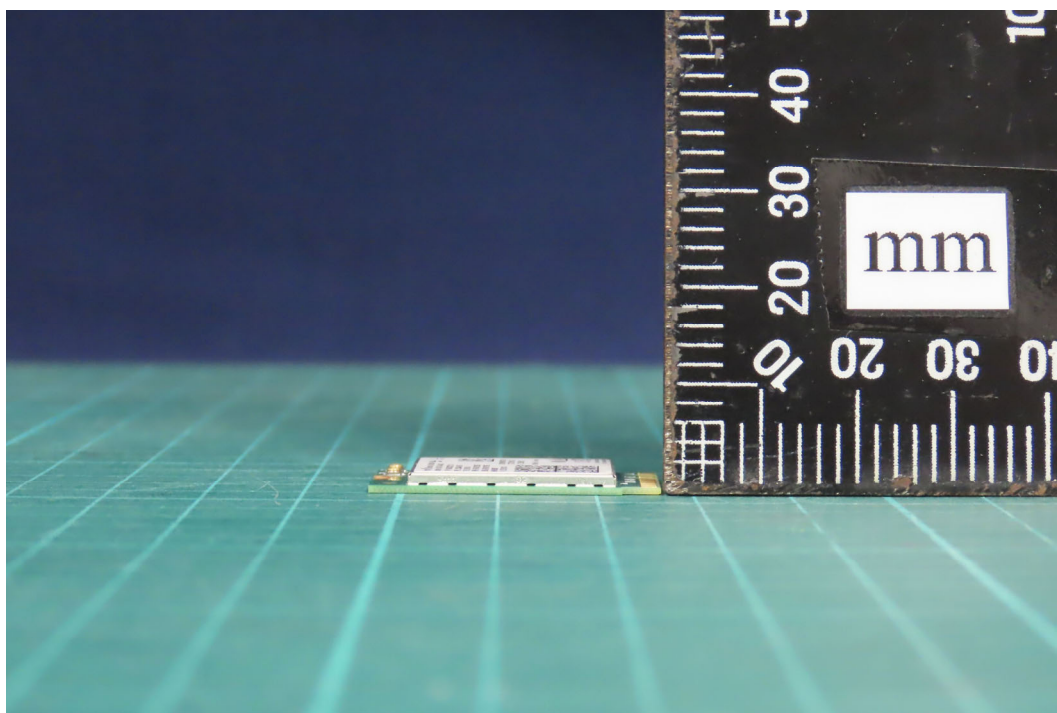
(74) EUT Photo
