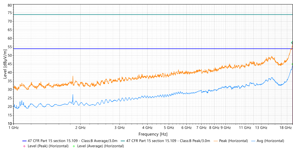
#1-1GHz-18GHz(Horizontal)
