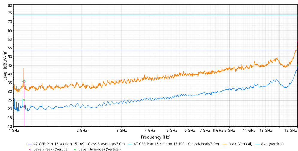
#2-1GHz-18GHz(Vertical)
