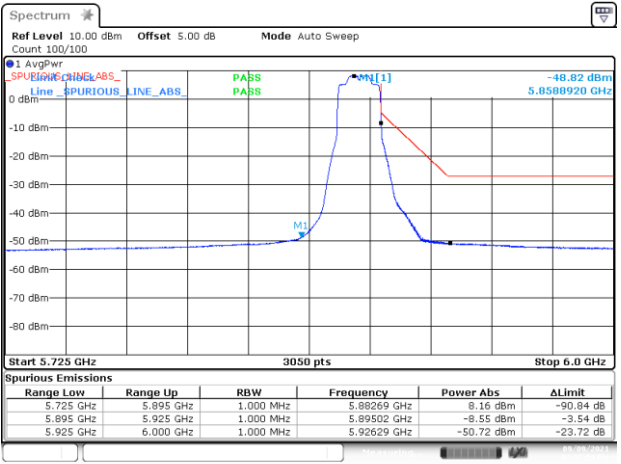
BE-NR-HIGH, MIMO-B, 802.11ax20-HE0, Ch177
