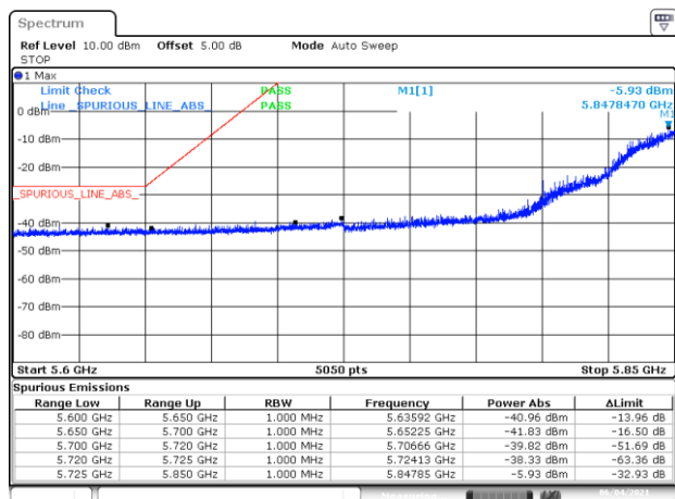
BE-NR-LOW, MIMO-A, 802.11n40-HT8, Ch175
