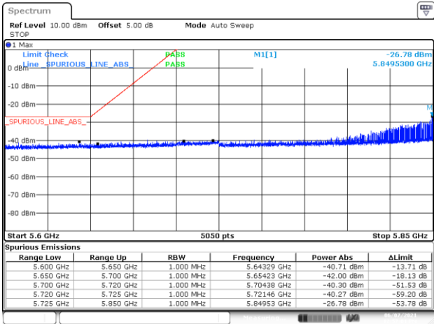
BE-NR-LOW, MIMO-B, 802.11ax20-HE0, Ch177
