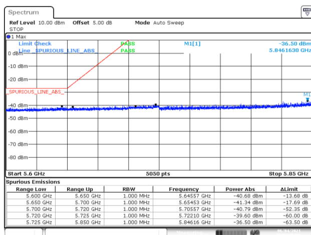
BE-NR-LOW, MIMO-A, 802.11ax20-HE0, Ch177
