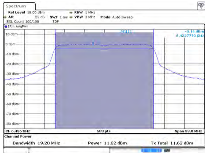
UNII-6 SISO B-802.11ax-20MHz-Ch97-6435MHz-MCS0
