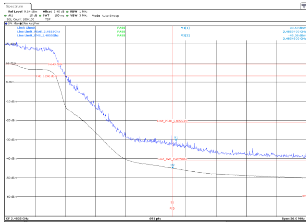
BE-R-HIGH, MIMO-A, 802.11ax20-HE0, Ch11
