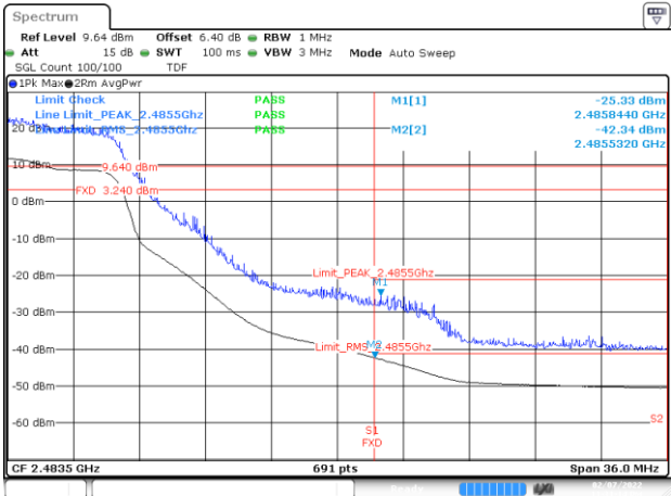
BE-R-HIGH, SISO-B, 802.11ax20-HE0, Ch11
