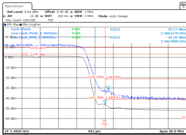
BE-R-HIGH, MIMO-A, 802.11ax20-HE0, Ch13
