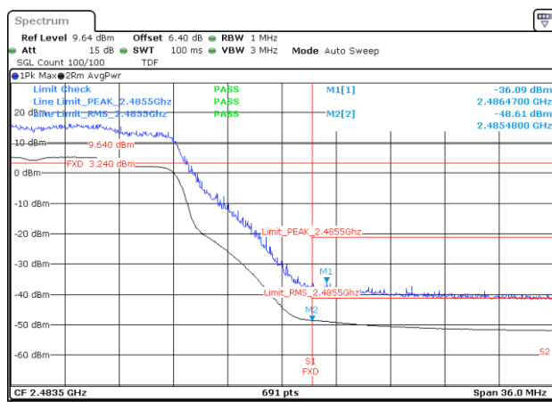
BE-R-HIGH, MIMO-A, 802.11ax20-HE0, Ch12
