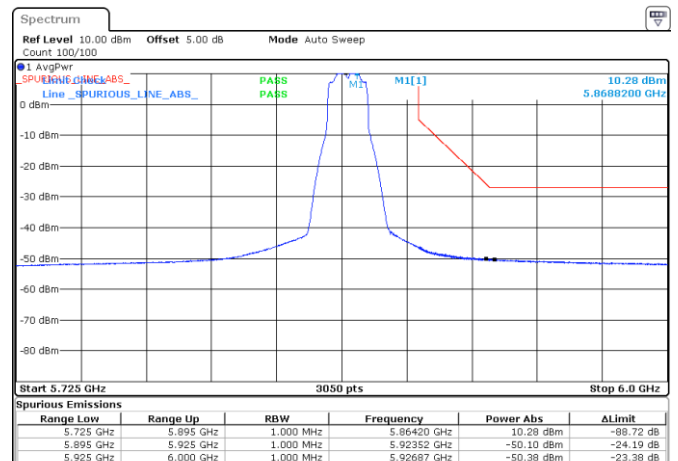
BE-NR-HIGH, SISO-A, 802.11a20-6Mbps, Ch173
