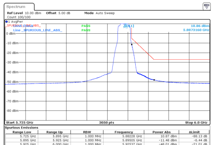
BE-NR-HIGH, SISO-A, 802.11a20-6Mbps, Ch177
