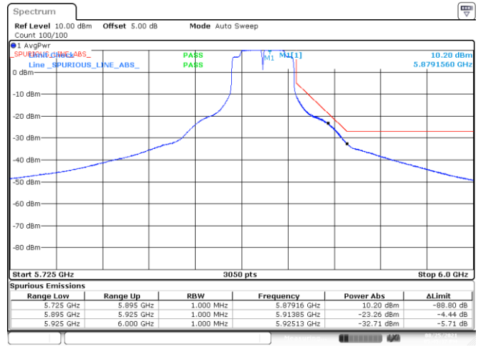
BE-NR-HIGH, SISO-A, 802.11n40-HT0, Ch175
