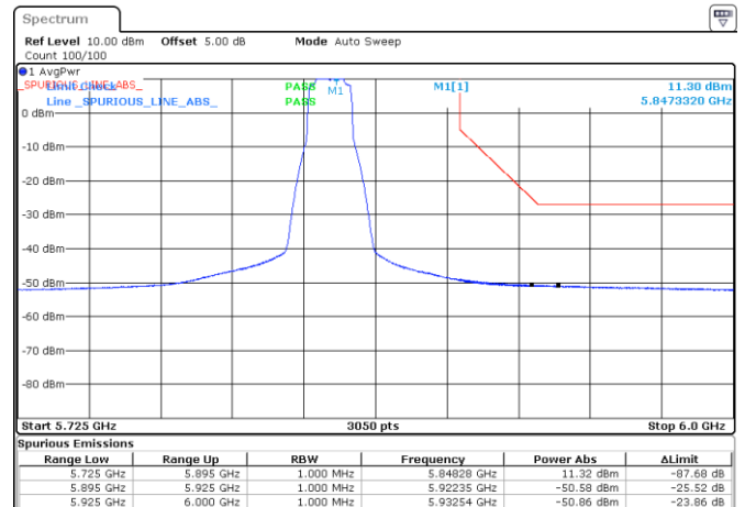
BE-NR-HIGH, SISO-A, 802.11a20-6Mbps, Ch169
