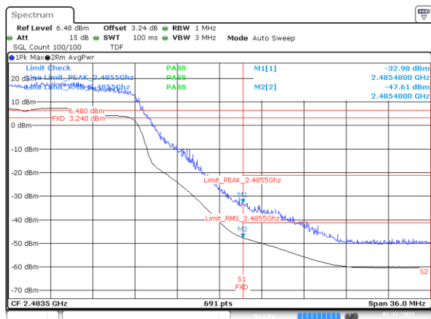
BE-R-HIGH, SISO-A, 802.11ax20-HE0, Ch12
