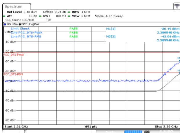
BE-R-LOW, SISO-A, 802.11ax40-HE0, Ch3
