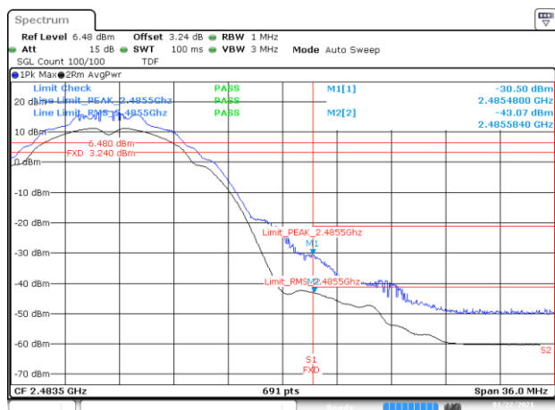
BE-R-HIGH, SISO-A, 802.11b-1Mbps, Ch13
