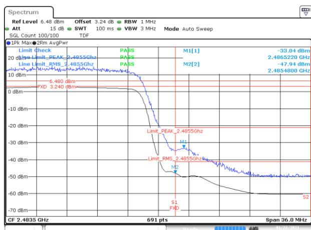
BE-R-HIGH, SISO-A, 802.11ax20-HE0, Ch13
