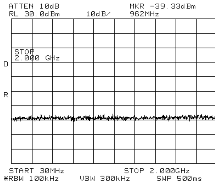
Spurious QPSK 30MHz – 2GHz, low
