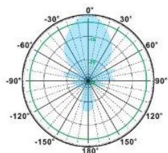
H-Plane
