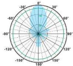
V-Plane
