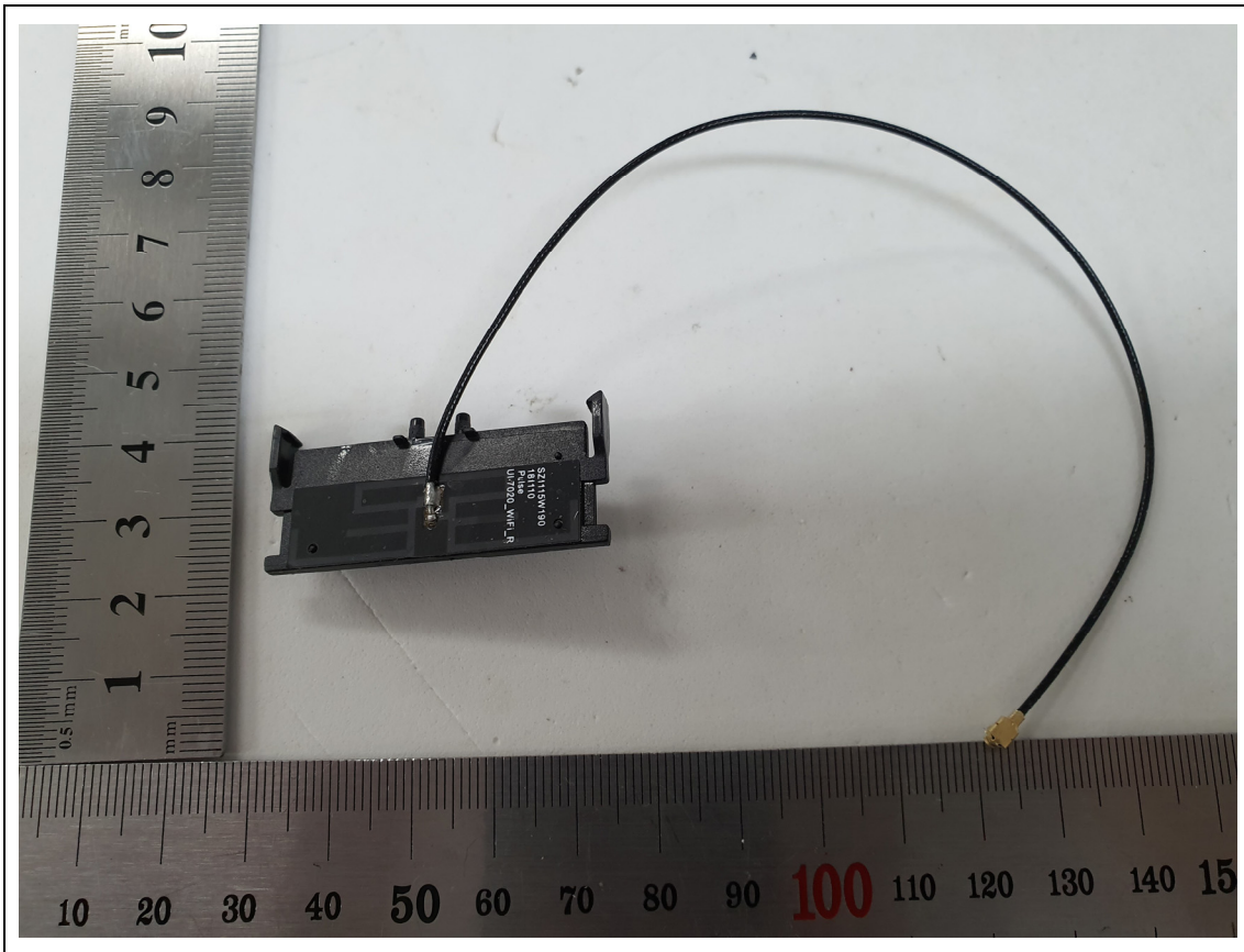
<Antenna 2>
