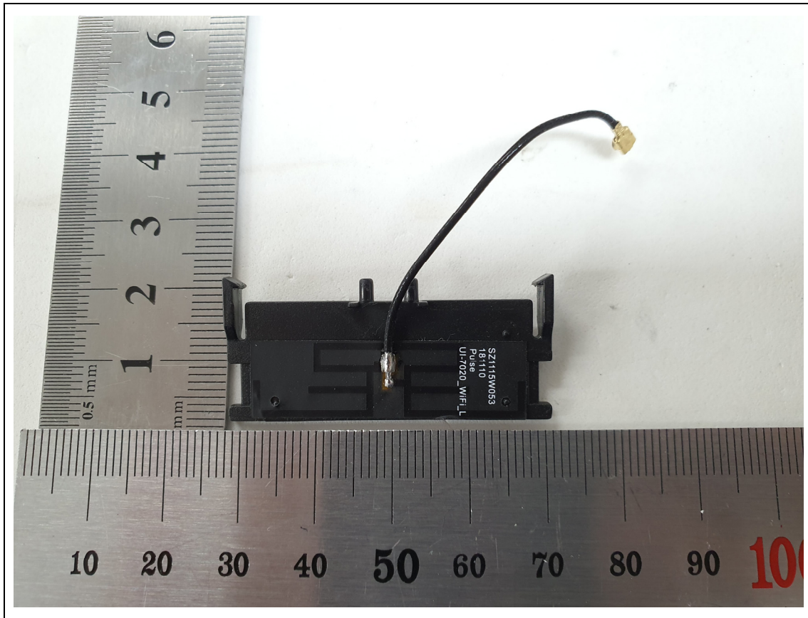
<Antenna 1>
