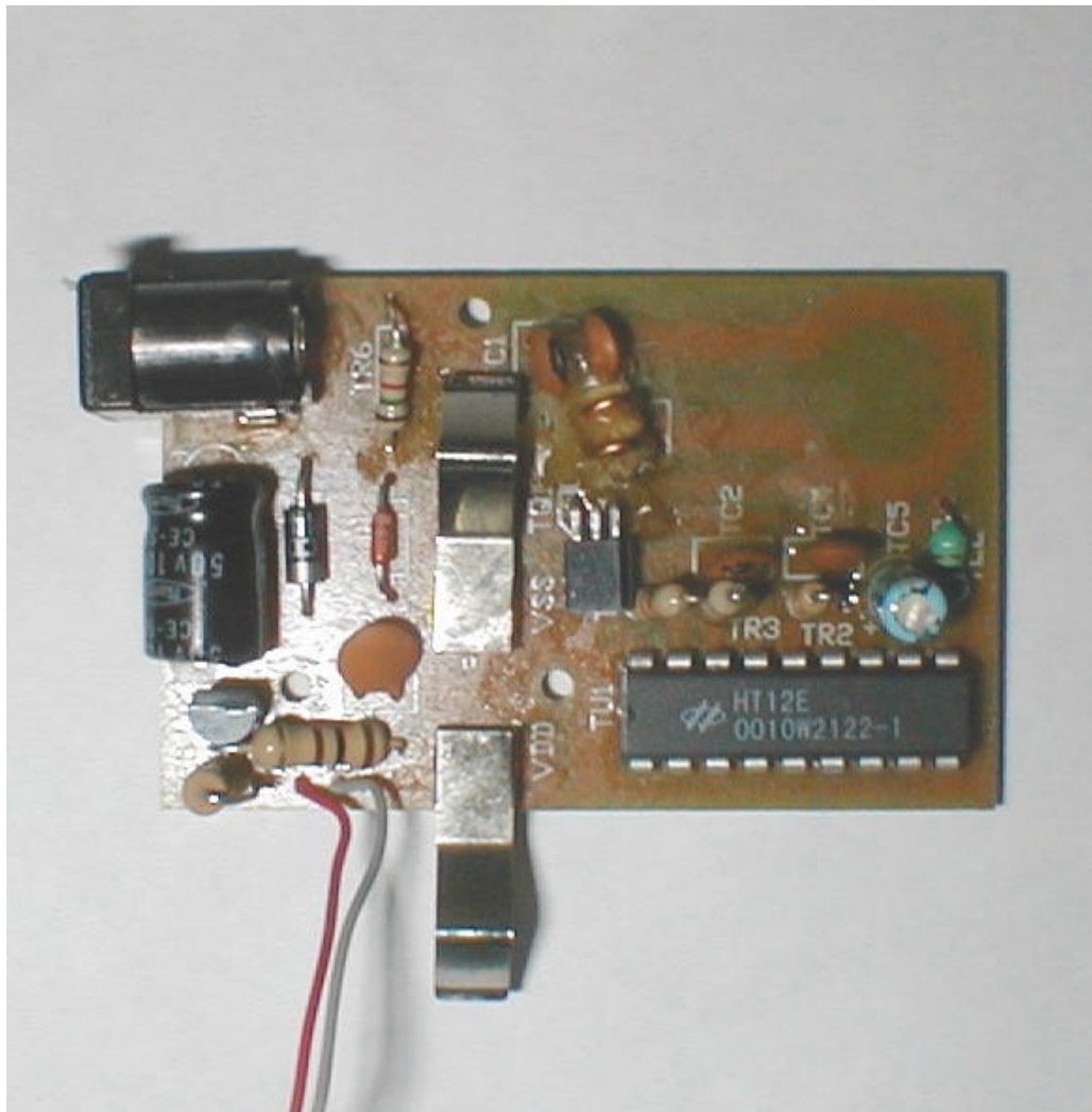
PCB Top
