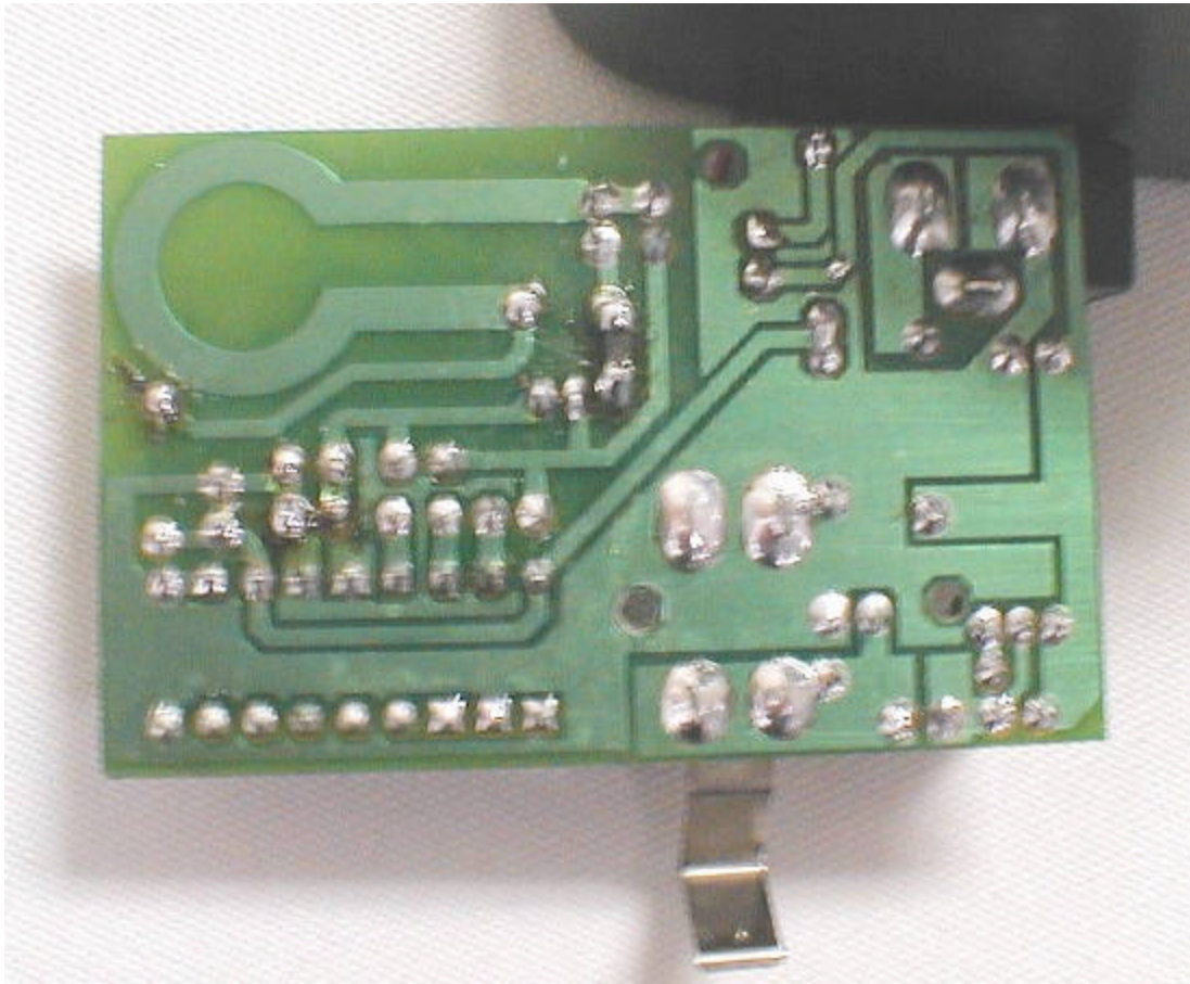
PCB Bottom
