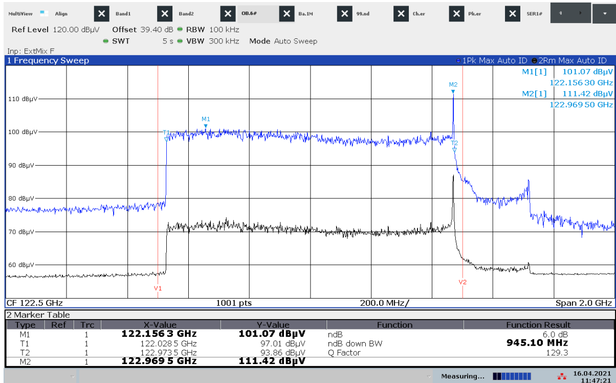
Plot 42: T_{\text{nom}} / V_{\text{min}}
