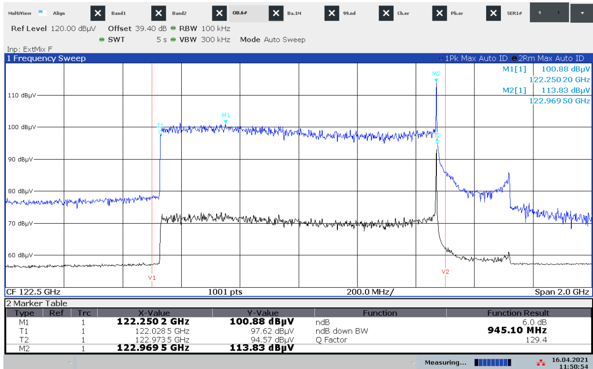
Plot 43: T_{\text{nom}} / V_{\text{max}}
