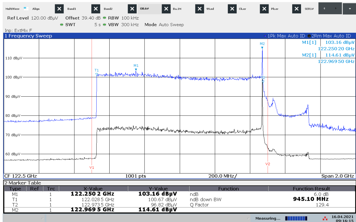
Plot 39: T_{nom} / V_{nom}
