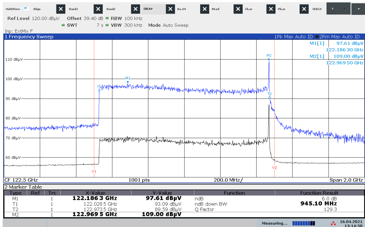
Plot 33: T_{nom} / V_{nom}
