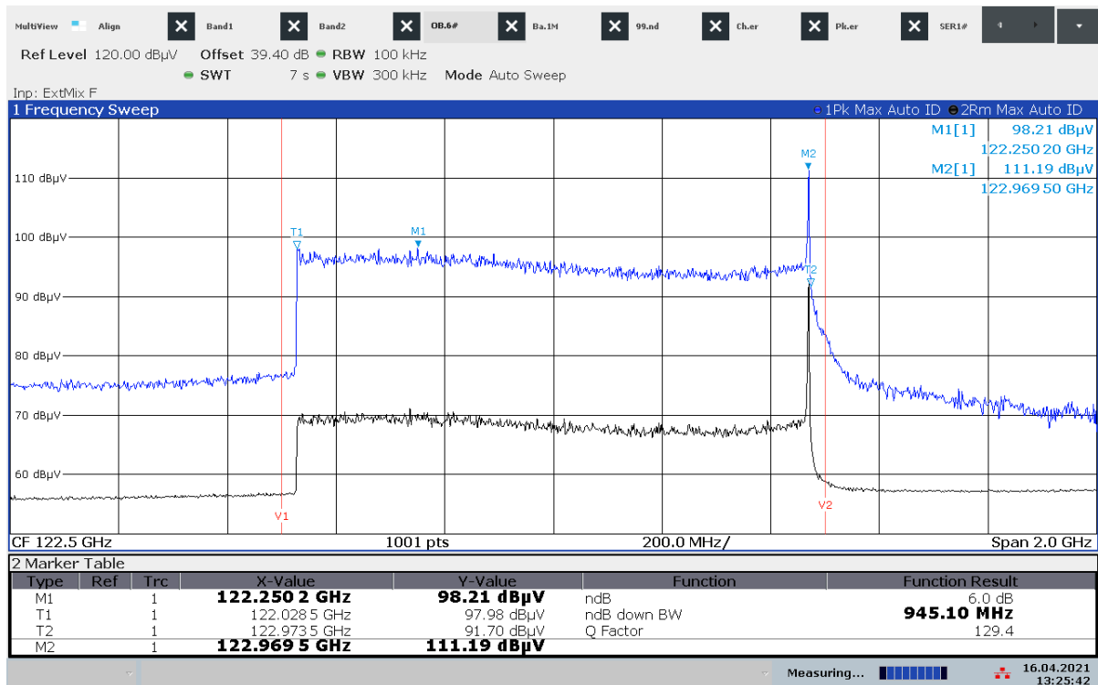
Plot 37: T_{nom} / V_{max}
