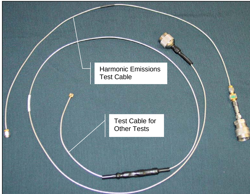
Test Cables
