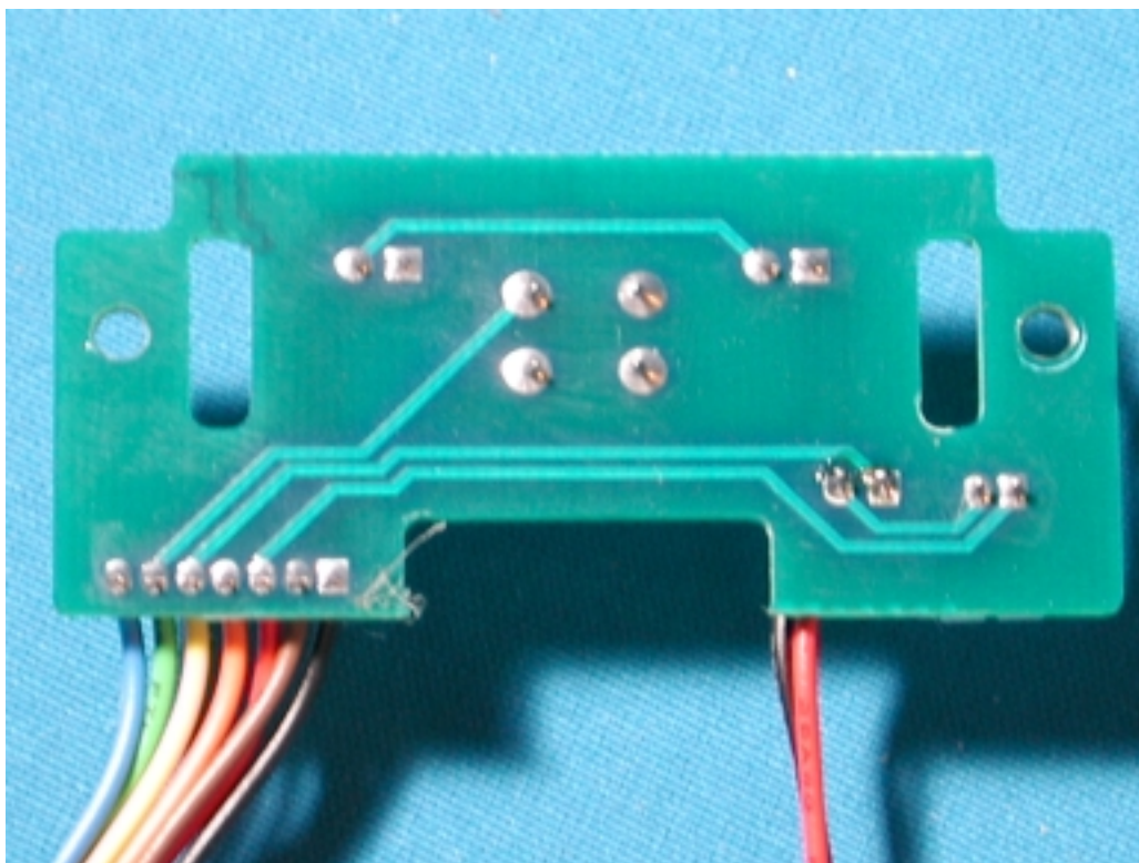
(9) EUT Photo
