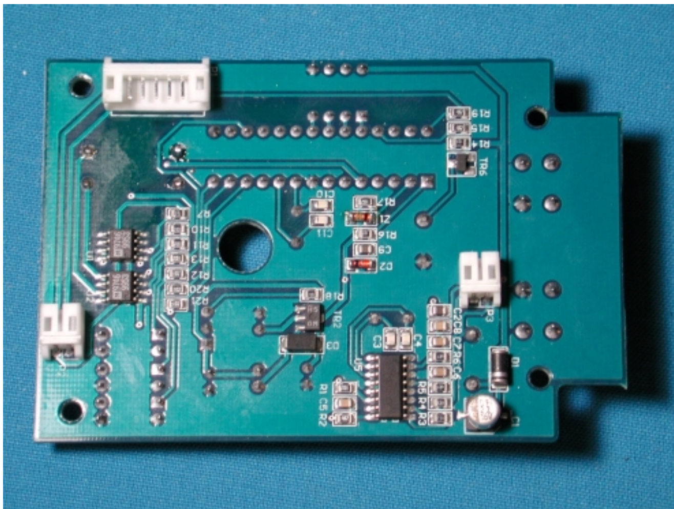
(13) EUT Photo
