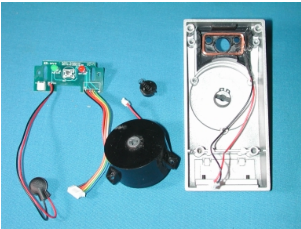
(6) EUT Photo
