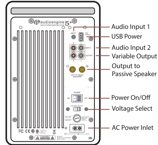
HD6 Back Left
