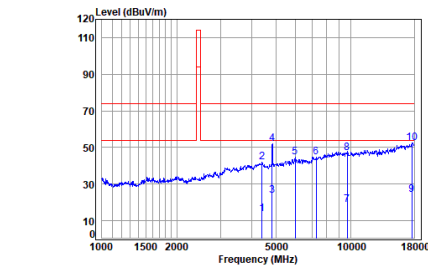
2.4G_SRD_LOW_TX_Horizontal
