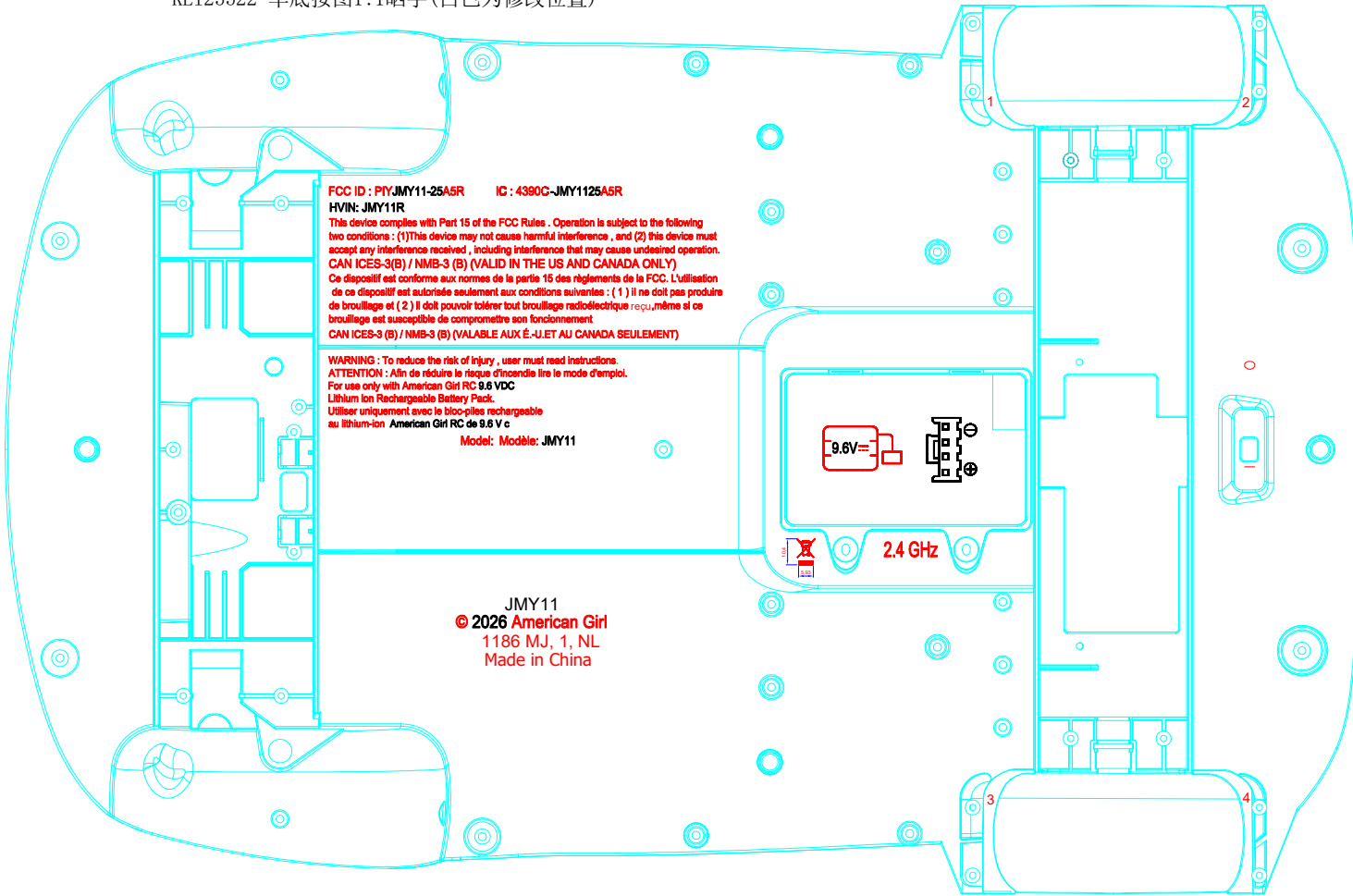
KL125522 车底按图1:1晒字 (白色为修改位置)
