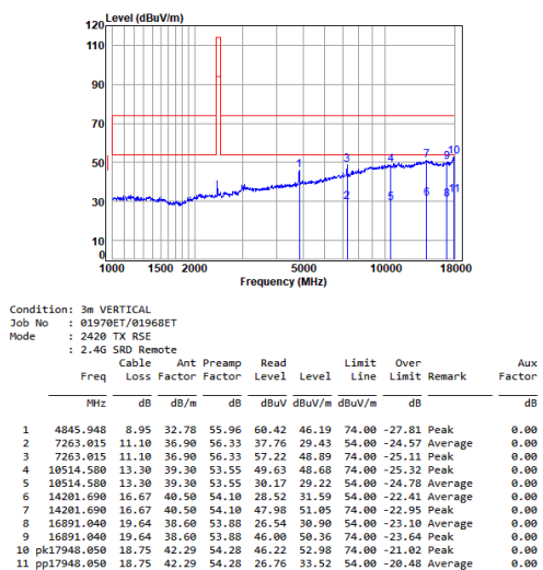
2.4G_SRD_TX_LOW_Vertical
