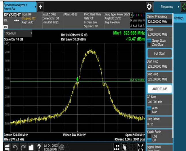
GPRS850-128
