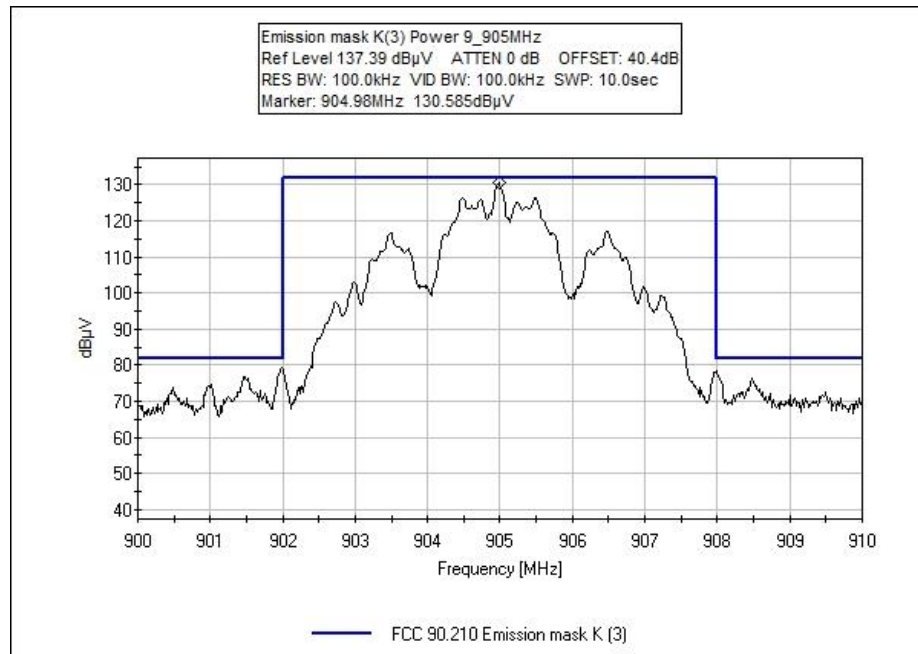
905MHz
