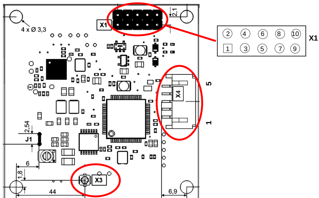
Abbildung 3 Überblick Anschlüsse und Stiftleisten
