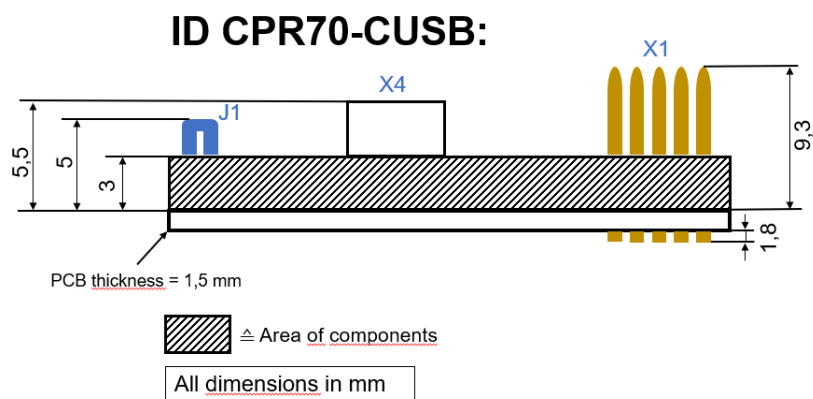
Abbildung 2: Bemaßung Vorderansicht Platine
