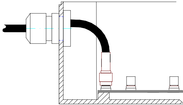
Bild 6: Readeranschluss
