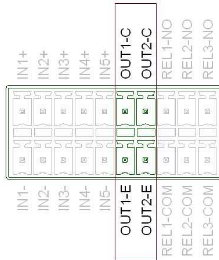
Fig. 15: Optocoupler -Outputs OUT1-2
