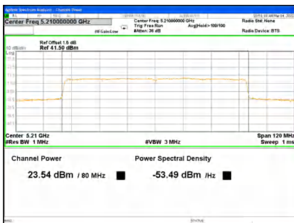
5210MHz_ax80_Ant B
