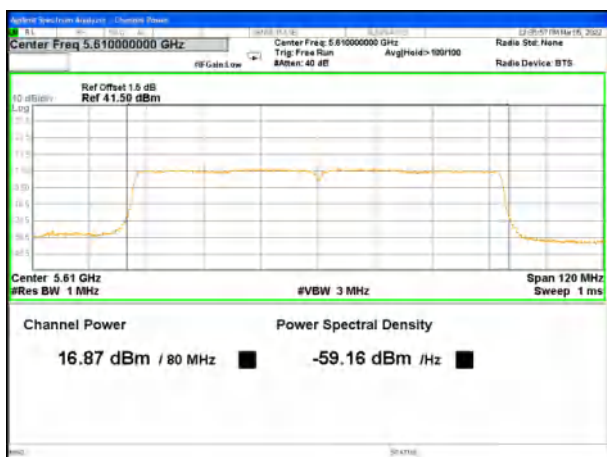
5610MHz_ac80_Ant A
