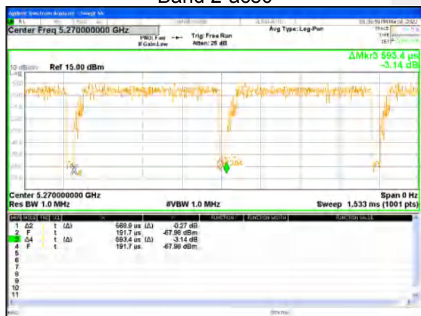
Band 2-ax40
