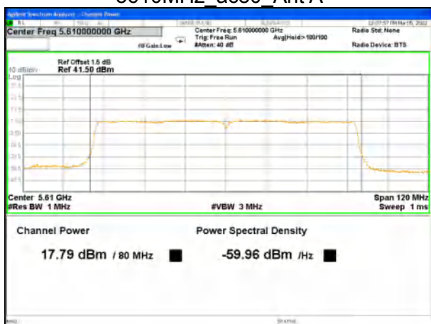
5610MHz_ax80_Ant A
