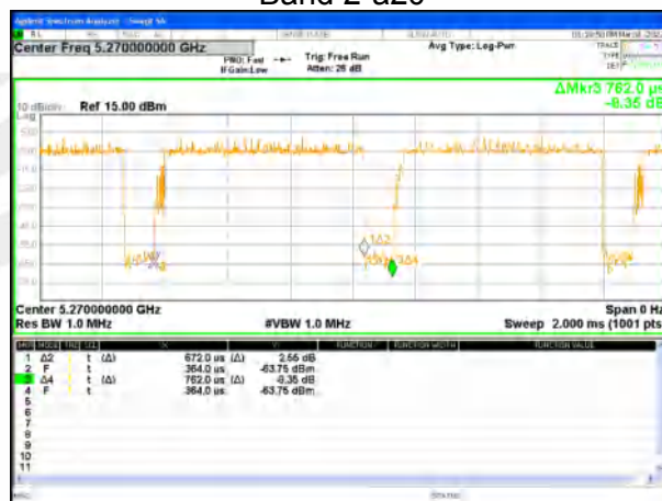
Band 2-n40
