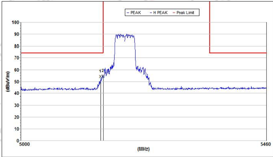
5210MHz Horizontal
