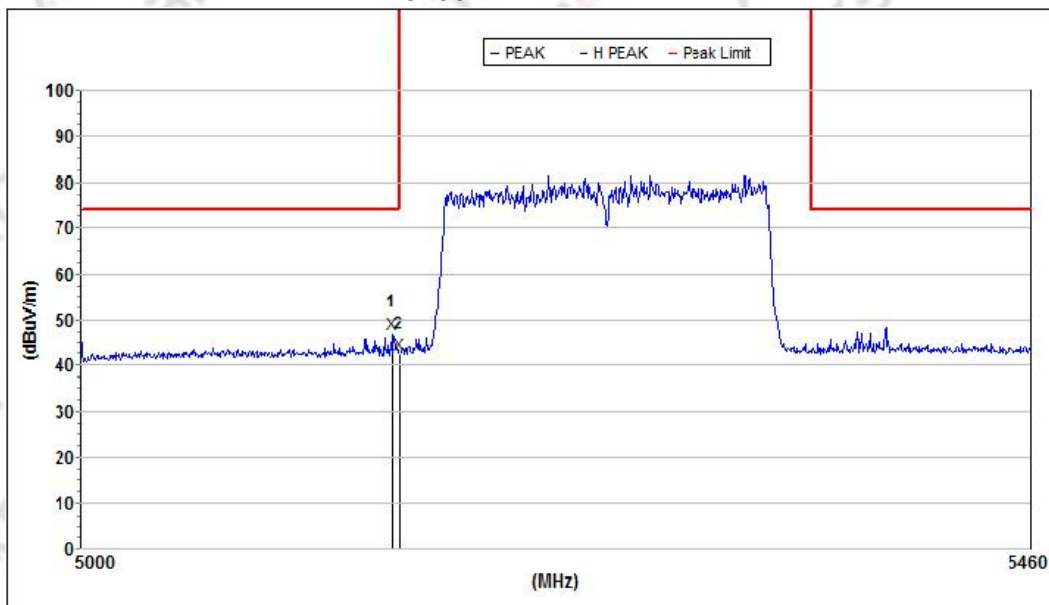
5250MHz Horizontal
